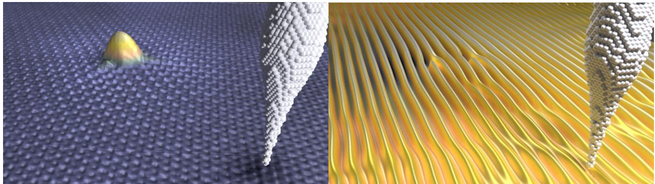
Figure 1 : En haut, une reconstruction 3D de l'image obtenue par microscopie à effet tunnel. On voit à droite de l'image une représentation artistique de la pointe qui sert à la mesure de cette image. Le dôme doré correspond à l'atome d'hydrogène. Les ondulations observées loin de cet atome proviennent du réseau atomique du graphène. D'autres oscillations liées à la réorganisation des électrons se superposent au voisinage de l'atome d'hydrogène. Ce signal est extrait et amplifié dans l'image du bas. On observe deux rangées supplémentaires dans les fronts d'onde : les dislocations. Ces dislocations sont la matérialisation dans l'espace réel de la singularité topologique du graphène.
