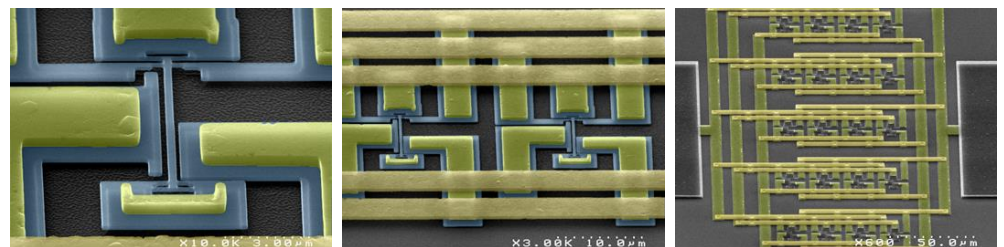
Photographies au microscope électronique d'un réseau de 20 nanorésonateurs en silicium connectés par des lignes métalliques, et zooms successifs sur un résonateur individuel (typiquement une dizaine de µm de long et une centaine de nm d'épaisseur).
