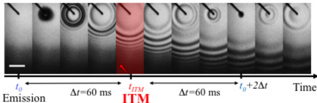
figure 1 : Dans le cas d'une perturbation ponctuelle, des ondes circulaires se propagent à la surface de la cuve. Après 60 ms, la cuve subit une accélération brutale de faible amplitude. Le paquet d'ondes initial se sépare en deux, avec une partie qui se reconcentre jusqu'à revenir à la perturbation ponctuelle (avant de se dissiper à nouveau). ©ESPCI Paris/CNRS
