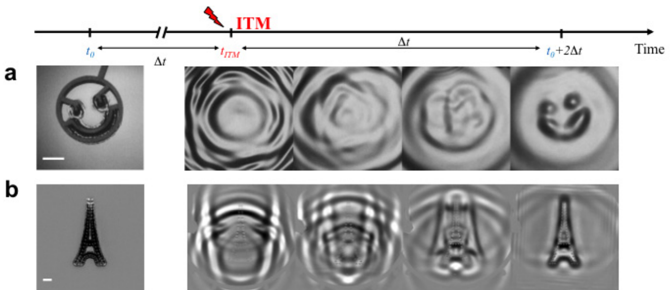
figure 2 : Dans le cas de systèmes complexes, la forme initiale de la perturbation est totalement perdue au moment de la brusque accélération de la cuve. Le retournement temporel instantané permet toutefois de bien revenir à la forme initiale du signal.
